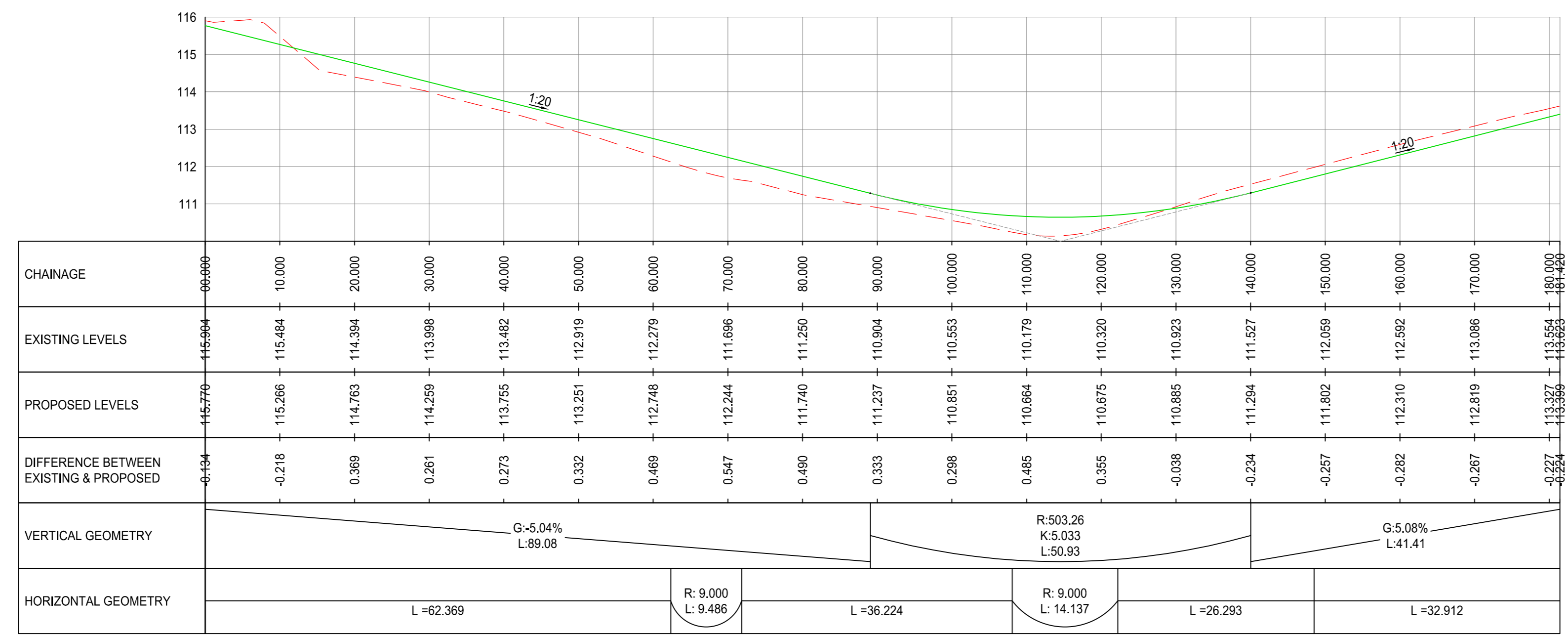
ALIGNMENT - (10) SCALE: H 1:500,V 1:100, DATUM: 110.000
