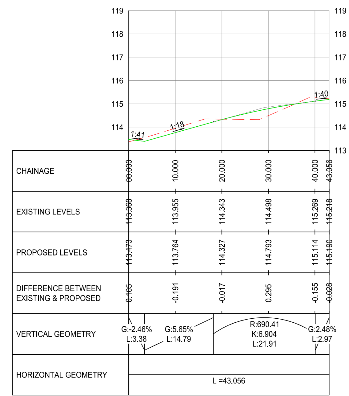
ALIGNMENT - (9) SCALE: H 1:500,V 1:100, DATUM: 113.000
