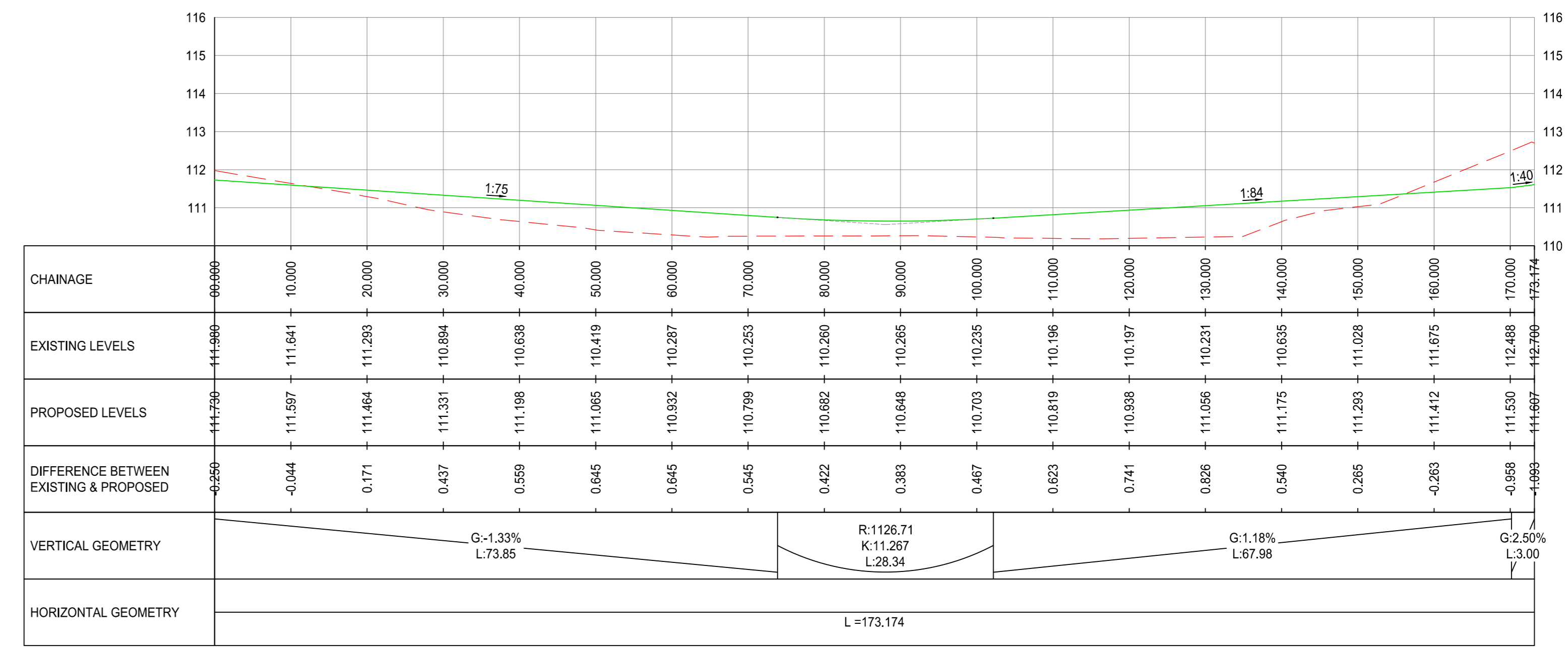
ALIGNMENT - (11) SCALE: H 1:500,V 1:100, DATUM: 110.000
